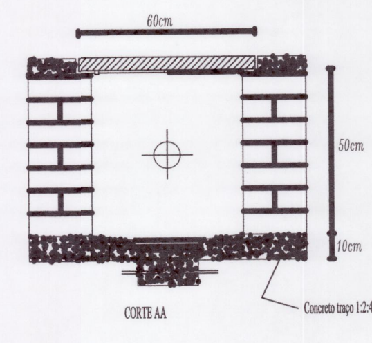
CAIXA SUBTERRÂNEA DE INSPEÇÃO P/ ATERRAMENTO
